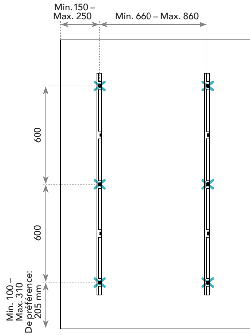
1760 x 1160 SCHÉMA DE LA PLAGE ACOUSTIQUE 6 spiral anchors per island
