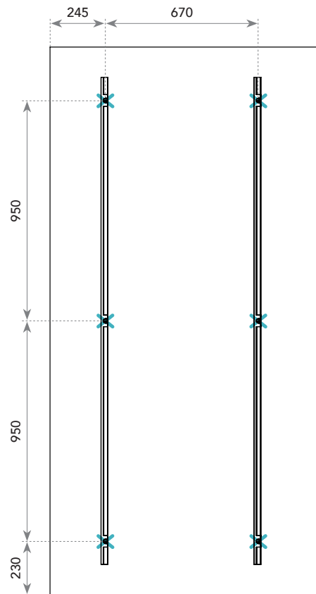
2360 x 1160 SCHÉMA DE LA PLAGE ACOUSTIQUE 6 spiral anchors per island
