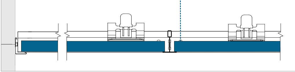
Bord A - Finition périphérique avec cornière de rive (profilé L) et clip anti-soulèvement.
