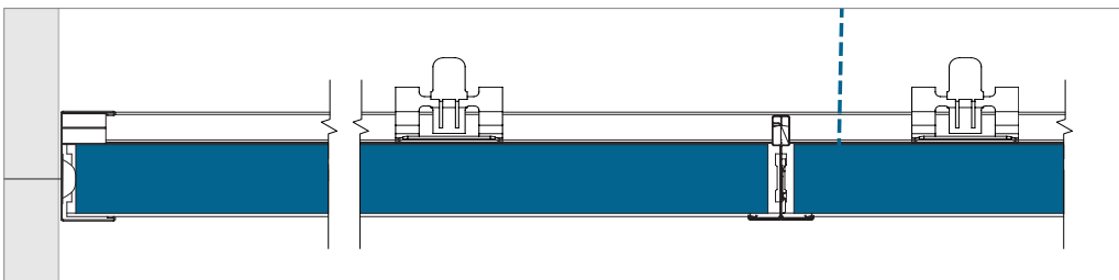
Finition périphérique avec coulisse de rive et clip anti-soulèvement.
