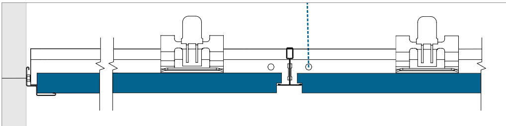
Bord E - Finition périphérique avec cornière de rive à joint creux et clip anti-soulèvement.
